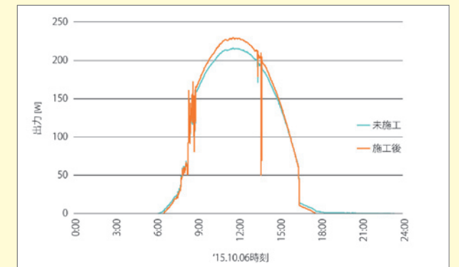
日中の出力推移
