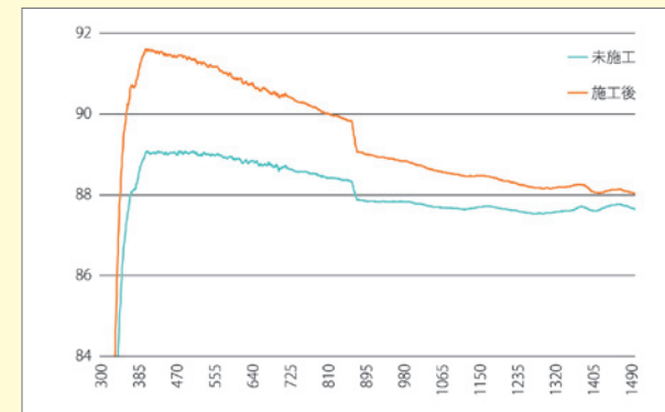
光の波長と透過率の関係
